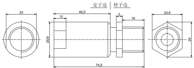
MSPS14A 尺寸图
