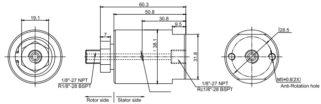
MSPS11A 尺寸图
