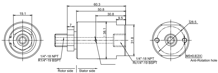
MSPS12A 尺寸图
