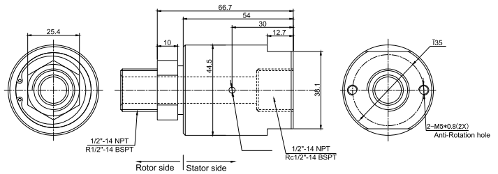
MSPS14 尺寸图
