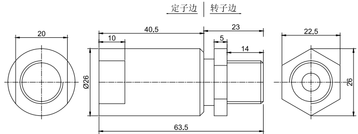
MSPS13A 尺寸图
