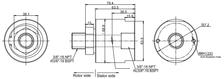
MSPS13A 尺寸图
