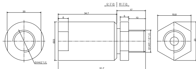
MSPS12A 尺寸图
