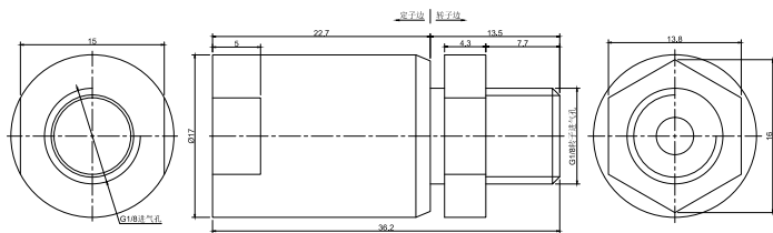
MSPS12 尺寸图
