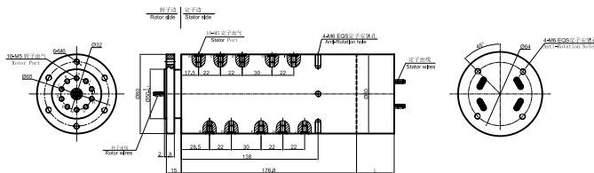
MAPH1000-01 尺寸图
